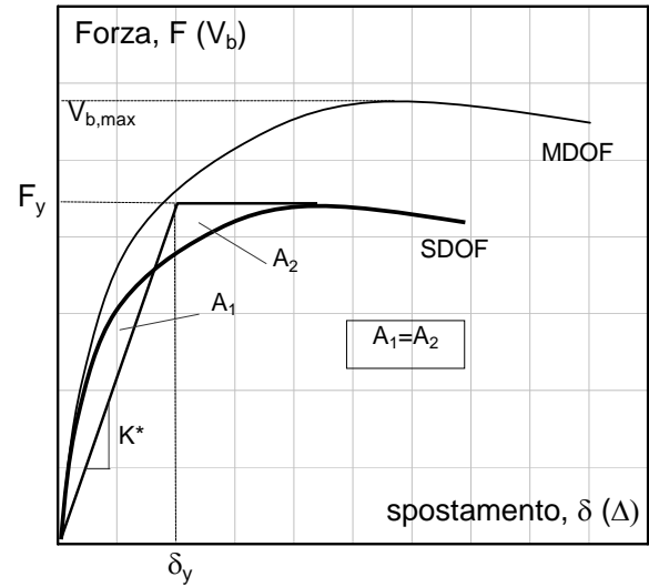
Figura 3. Rappresentazione elasto-plastica della curva di push-over
